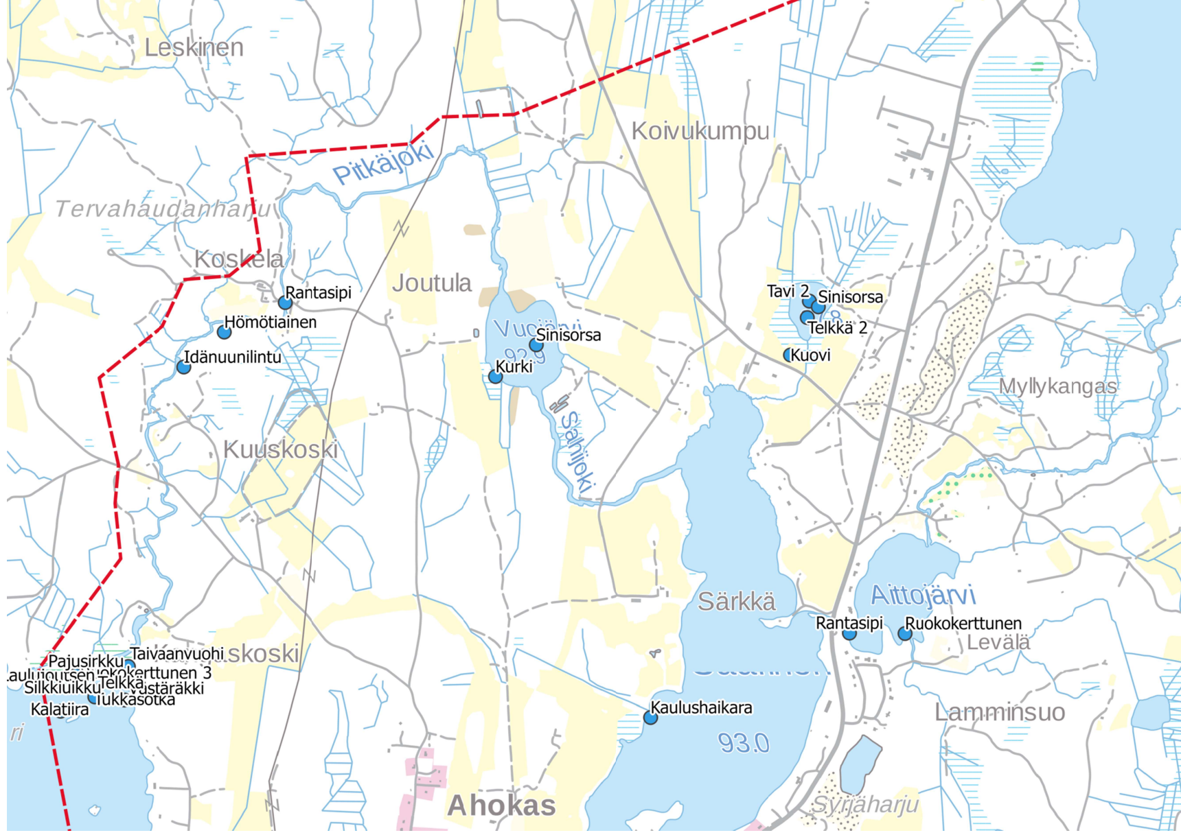
Kuva 3. Selvitysalueen pohjoisosat.
