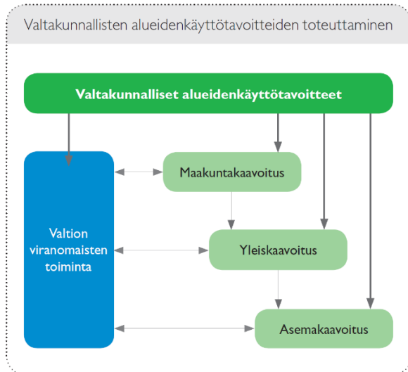
Kuva 19: Kaavahierarkia
